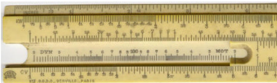
afb. 3 – onder de schuif: deel 20 – 200 van C-schaal
