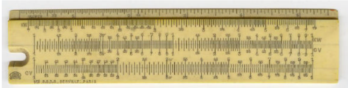
afb. 1 – Voorzijde: 5½ in / C 736 (KW) – A (KW) = B (CV) – C = D (CV)
